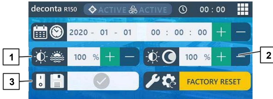
Abb. 18 Button „Displayhelligkeit“
